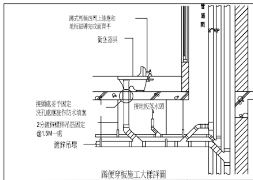
蹲便穿板施工大樣詳圖
