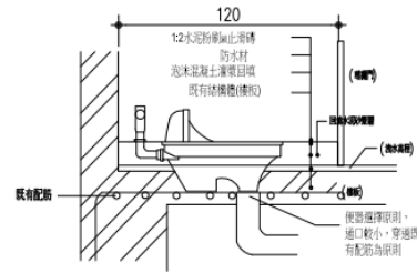
蹲便施工大樣詳圖
