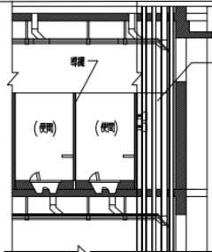
便器與管道剖面詳圖
