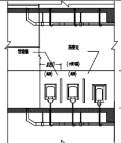
便器剖面詳圖
